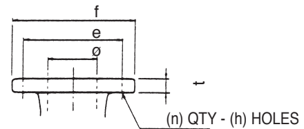
Flange (ANSI 125 PSI F.F)
